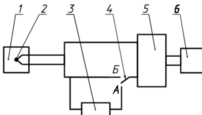
Рисунок 1 — Структурная схема измерения температуры без градуировки измерительного тракта
