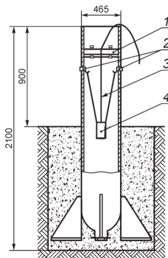
Рисунок 4б – Схема эффектомера 5 \text{ м}^3
