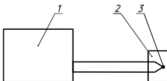
1 — потенциометр КСП; 2 — испытуемое ПИ; 3 — термообразователь
